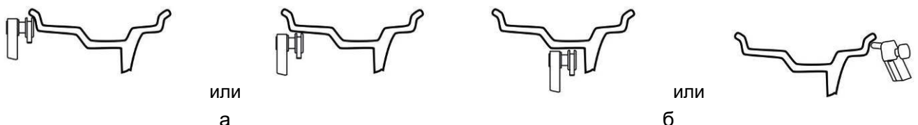
Рисунок 5.10 – Подвод линейки при прямом измерении
