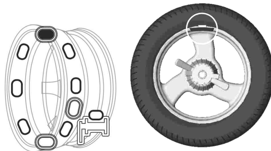
Рисунок 6.3 – Груз установлен в положение «12 часов»
