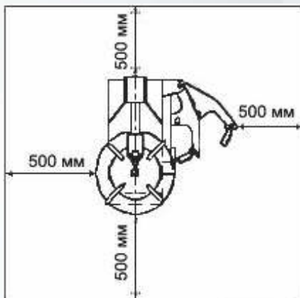
Рисунок 4.1 Установка стэнда
