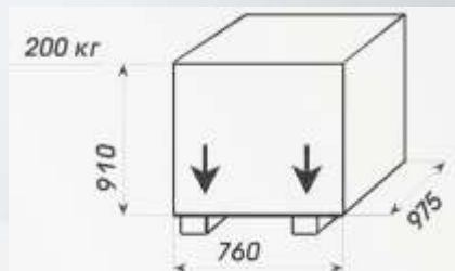
Рисунок 3 Габаритные размеры
